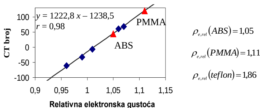
Slika 3. Linearni odnos CT-broj – relativna elektronska gustoća. Plavi kvadratiči predstavljaju 5 tkivo-ekvivalentnih umetaka u CIRS fantomu, koji određuju pravac linearne regresije y = 1222,8x - 1238,5 pomoću kojeg je izračunata relativna elektronska gustoća ABS, PMMA fantoma i teflona.
