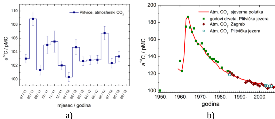
Slika 1. a) a^{14}\text{C} u mjesečnim uzorcima atmosferskog \text{CO}_2 na području Plitvičkih jezera u razdoblju 2011. – 2012. b) Prosječne godišnje vrijednosti a^{14}\text{C} atmosferskog \text{CO}_2 te a^{14}\text{C} u godovima drveća s područja Plitvičkih jezera za razdoblje 1950. – 2010. [1,3].
